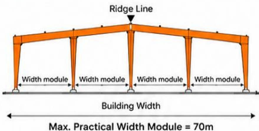
MULTI SPAN "3" (MS-3)
