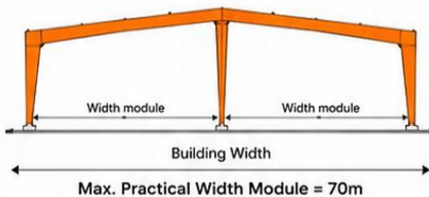
MULTI SPAN "1" (MS-1)
